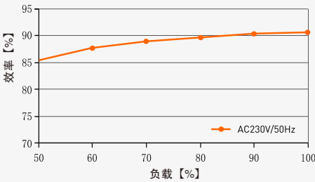
效率与负载关系图表
